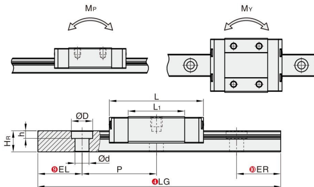
4-1 DGMN系列-微型滚珠直线导轨
