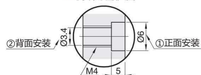
★ ⑤ 安装孔放大图
