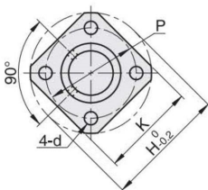
方法兰型
