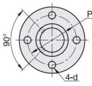
圆法兰型
