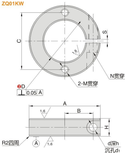
微调整环 ZQ01KW
