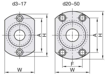
对边法兰型
