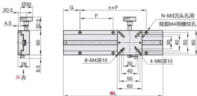
ZD50LB-L400
