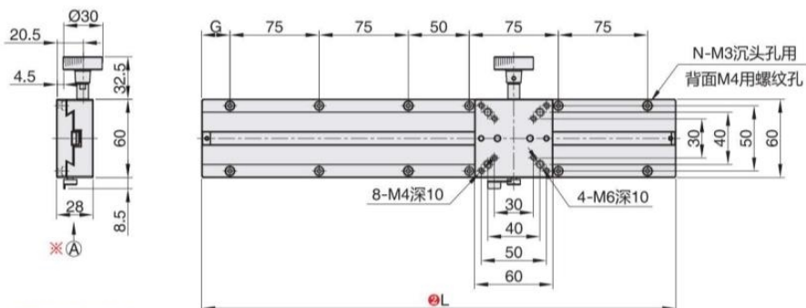
ZD50LB-L500
