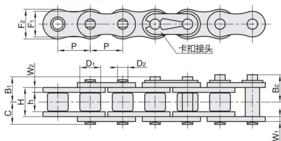
链条 CD30GE/CD31GE
