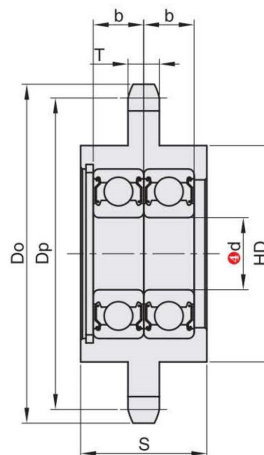
双轴承 CD23BF
