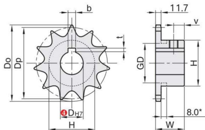
链轮 CD21EF/CD21EU
