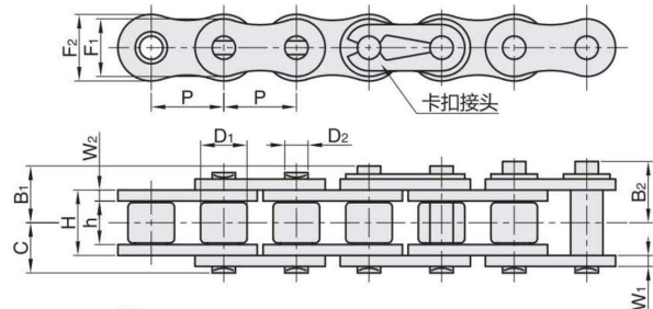
链条 CD30EE/CD30EU/CD31EE
