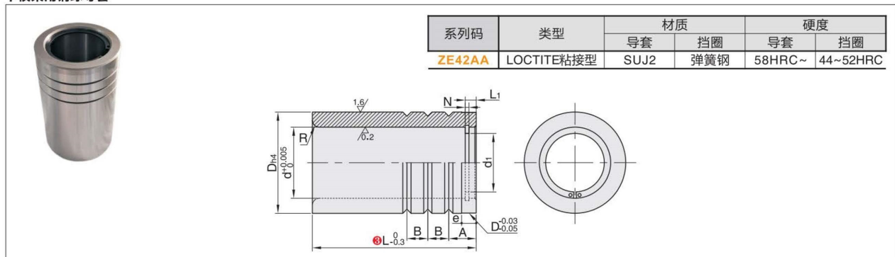
下模架用钢球导套
