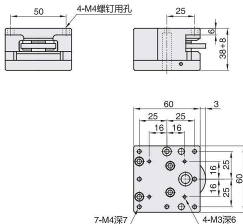
进给丝杆驱动型 ZD49JB-60
