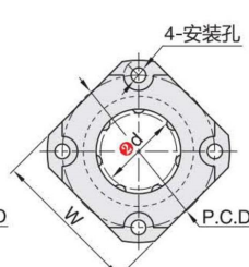
方法兰型
