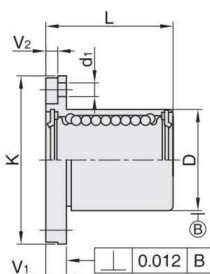
单衬型
