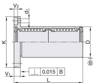
单衬型
