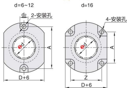
对边法兰型
