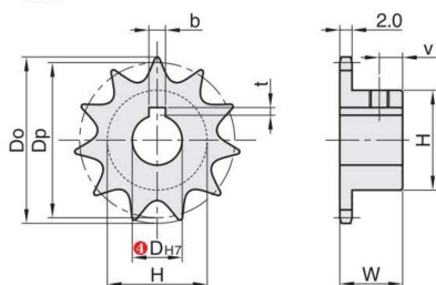
链轮 CD21HF
