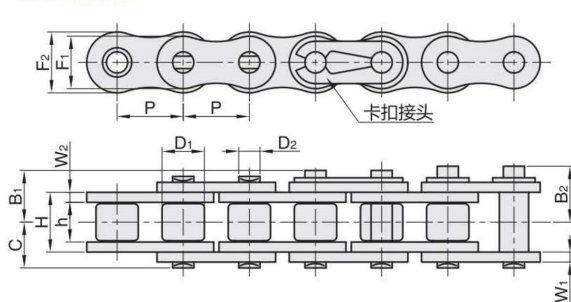
链条 CD30HE
