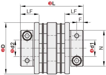
QLTSF(双膜片型) 外径 \varnothing 56 \sim \varnothing 82
