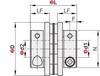
QSTS(单膜片型) 外径 \varnothing 56 \sim \varnothing 82
