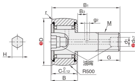
圆弧型•带密封圈型 CA76DS/CA76DH
