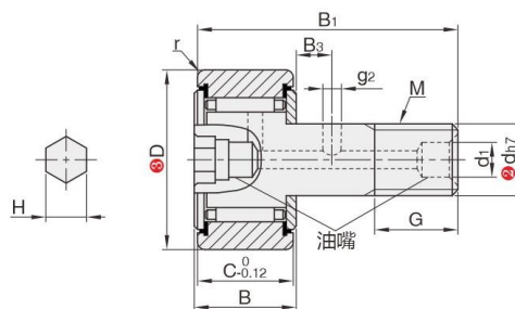
圆柱型•带密封圈型 CA76BS/CA76BH
