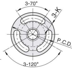
腰孔型
