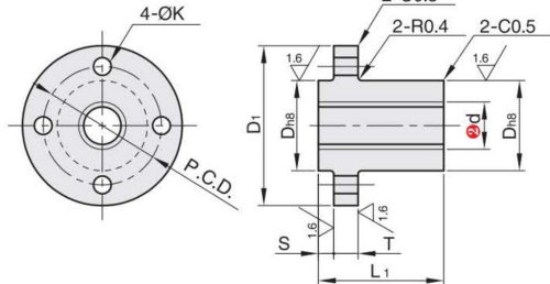
嵌入型
