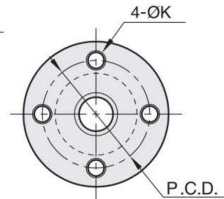
螺孔型
