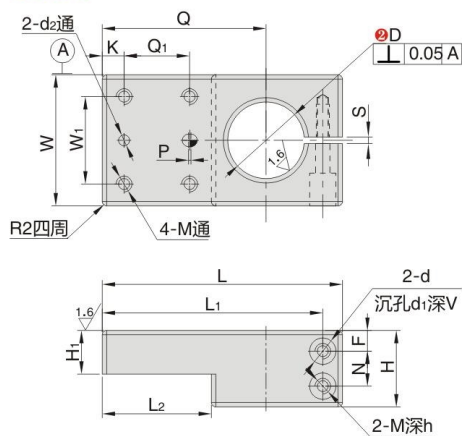
平行锁块 ZQ01FW
