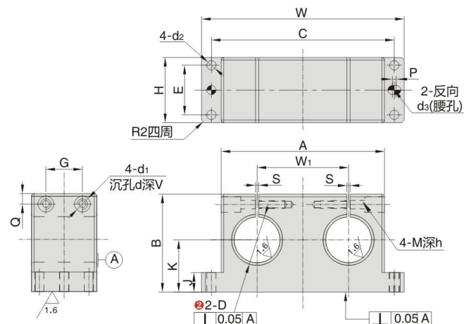
双孔锁块 ZQ01HW
