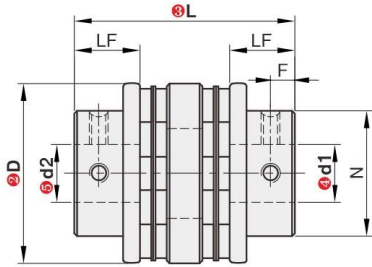
QLMTSF(双膜片型)
