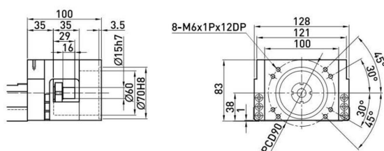
电机连接法兰MKK130-F2
