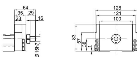
转接固定座MKK130-H0
