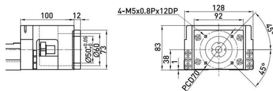
电机连接法兰MKK130-F3 (86步进电机)
