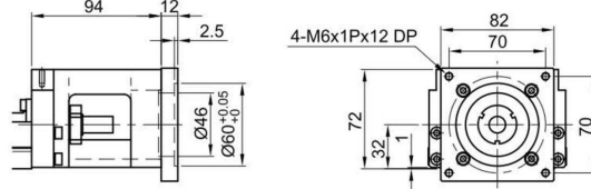
电机连接法兰 MKK100-F3
