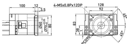
电机连接法兰MKK130-F4 (松下750W)
