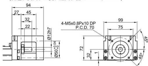
电机连接法兰MKK100-F2 (松下750W)
