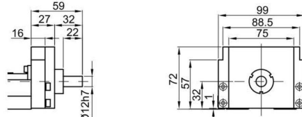
转接固定座 MKK100-H0
