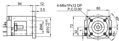
电机连接法兰 MKK100-F3
