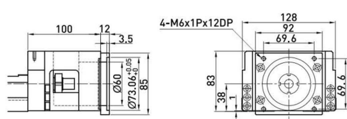
电机连接法兰MKK130-F3 (86步进电机)
