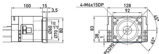
电机连接法兰MKK130-F4 (松下750W)
